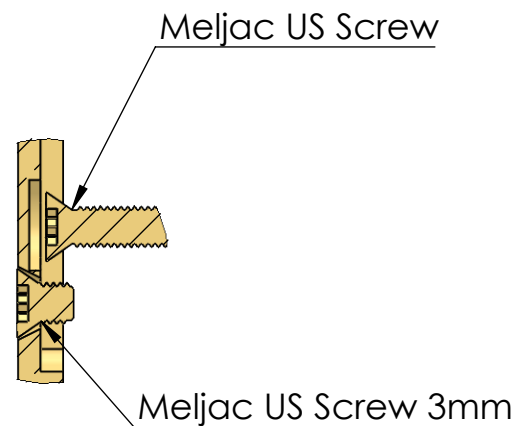
DÉTAIL C ECHELLE 6 : 4
